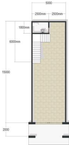
Lantai I
